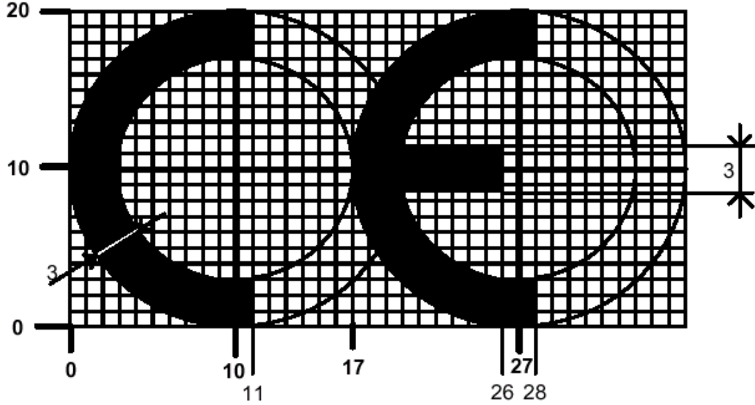
Şekil-1 CE işaretinin ölçüleri
