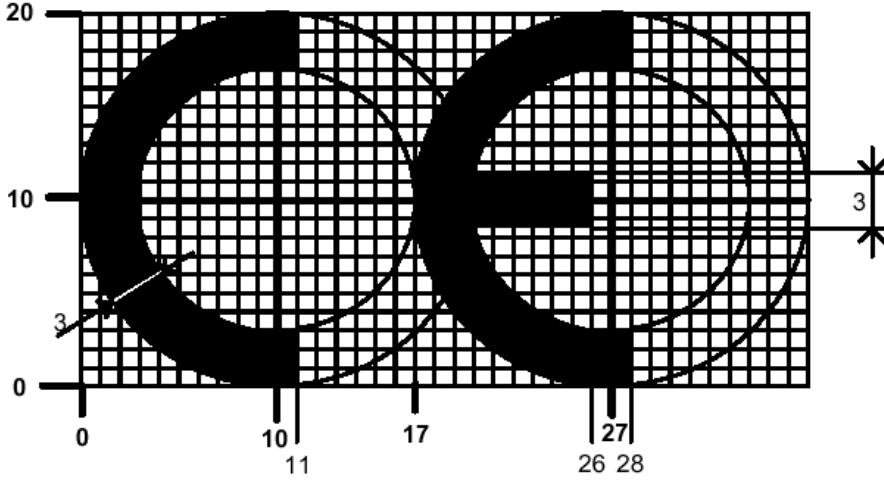
Şekil-1 CE işaretinin ölçüleri
