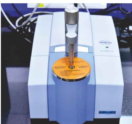
FTIR
